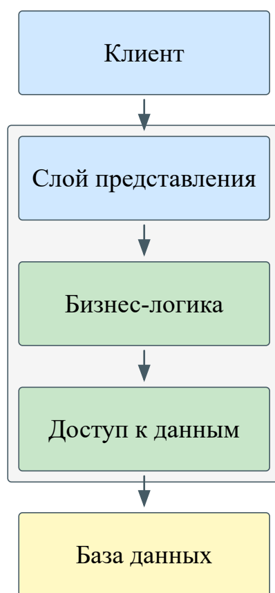
Рис. 5. Монолитная архитектура
