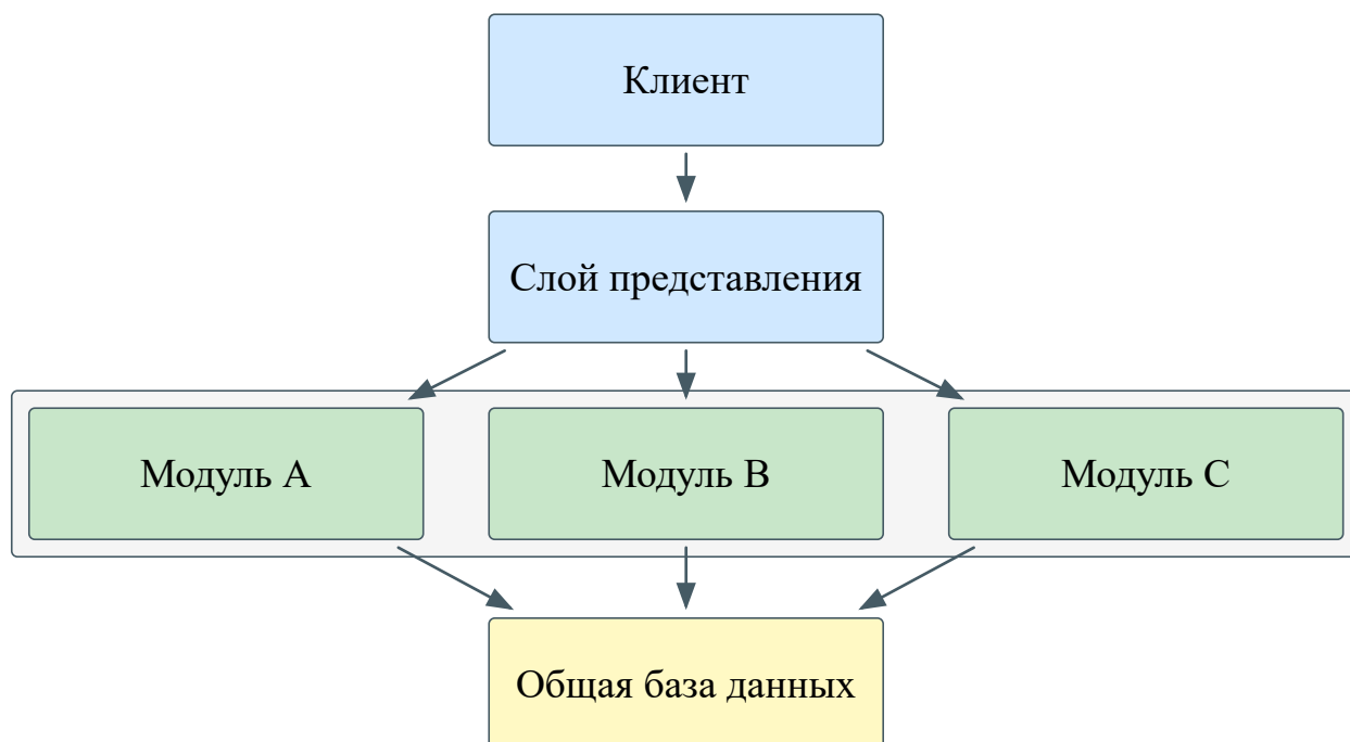
Рис. 7. Модульно-монолитная архитектура
