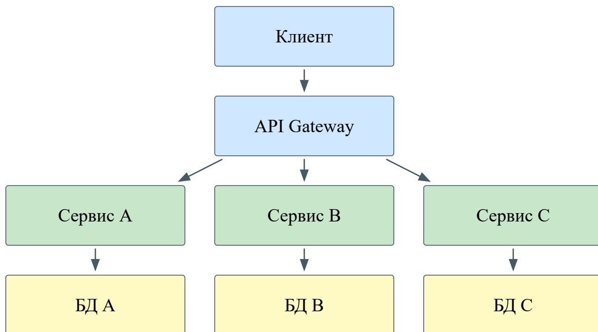
Рис. 6. Микросервисная архитектура
